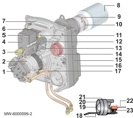
Abb.3 Hauptkomponenten
