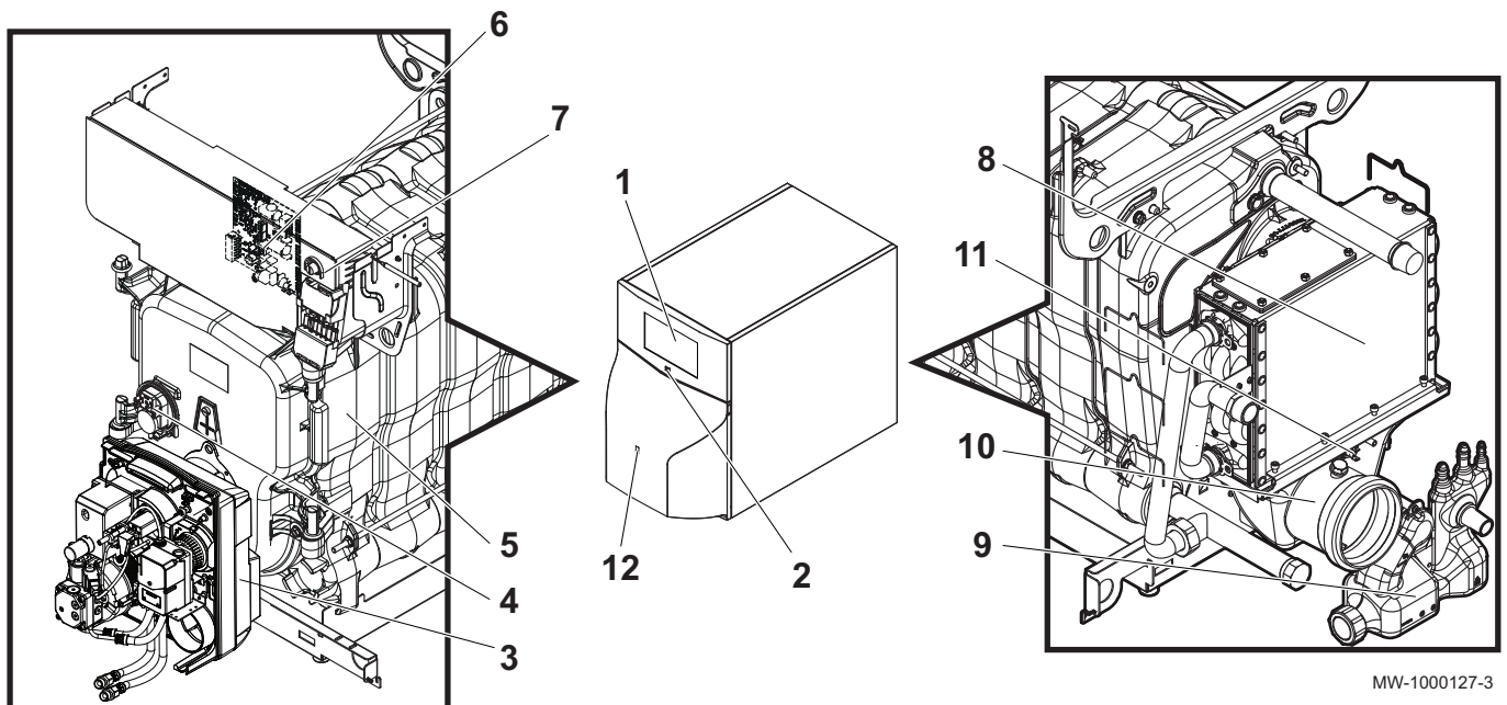
Abb.2 Hauptkomponenten
