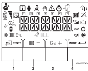
Abb.6 Tasten der Bedieneinheit
